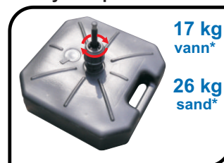
Fyllbar plastfot
